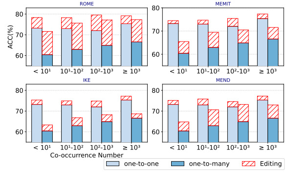
(b) Llama2
