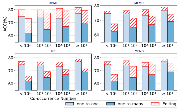
(a) Llama3
