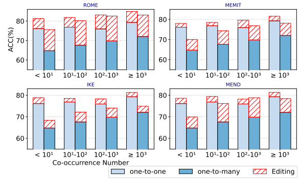
(b) Qwen2.5
