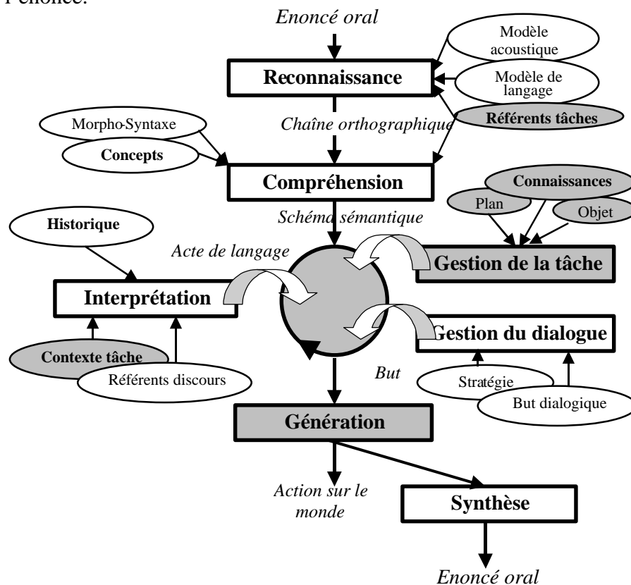
Figure 1 : Architecture générique d'un système de dialogue homme-machine, les parties grisées correspondent aux connaissances ou traitements dépendants de l'application
