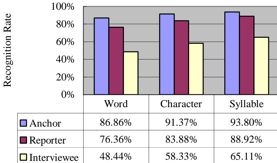
圖六、加入語言模型及音節間靜音長度後之語音辨識率。
