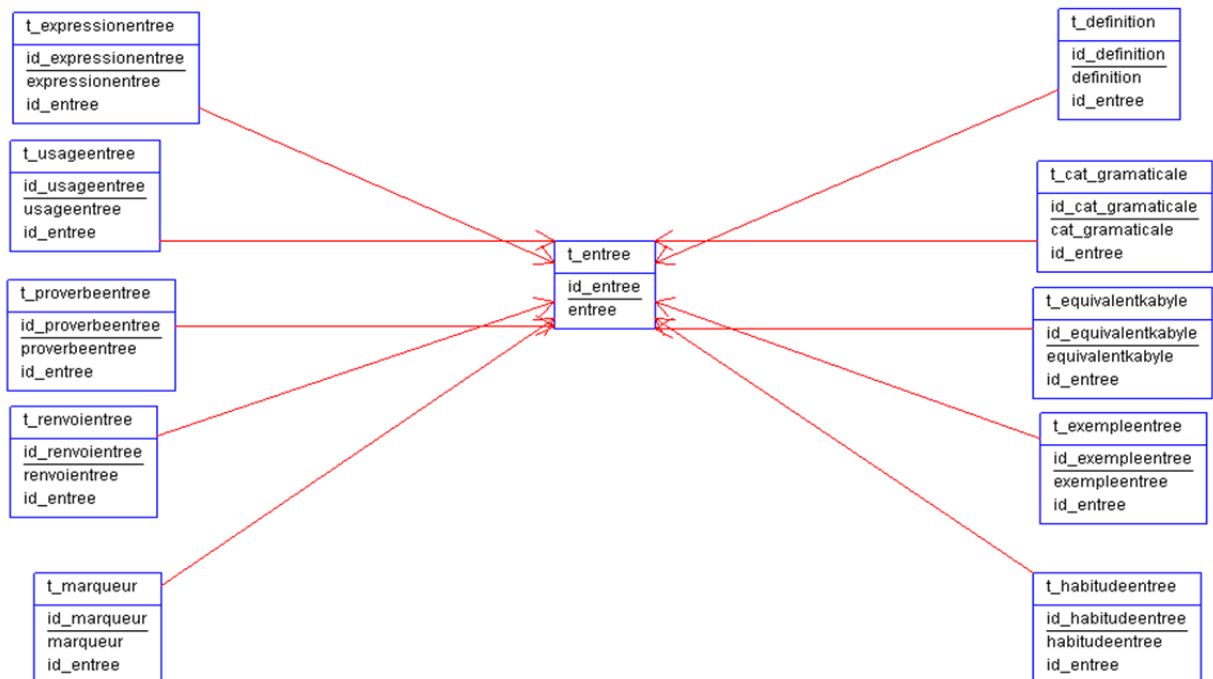
Figure 4. Schéma conceptuel MLD.
