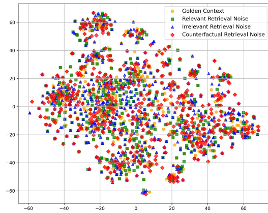
a) \mathbf{RALM}_{golden}
