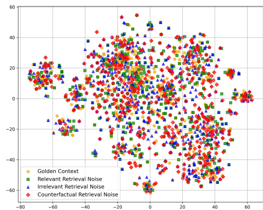
b) \mathbf{RetRobust}
