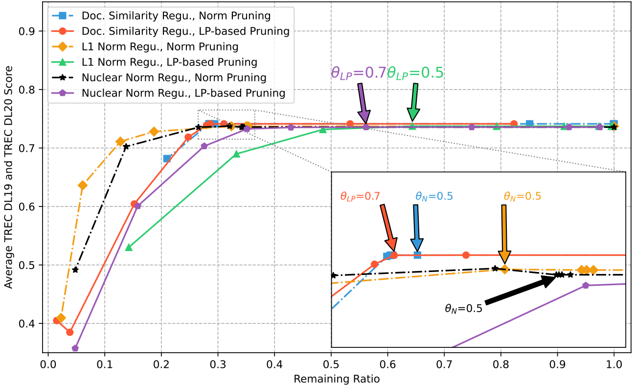
FIGURE 2 – Moyenne de TREC DL (2019 et 2020) nDCG@10 pour différentes régularisations et ratios d’élagage.
