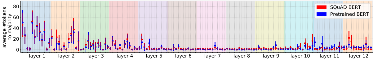
(b) BERT
