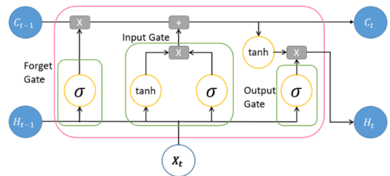
圖 1: LSTM 模型的示意圖。
