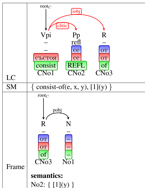
Figure 11: Lexical Entry for състоя се от “sastoya se ot”, ‘I consist of’.
