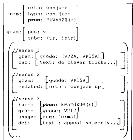
Fig. 15. Overriding of values
