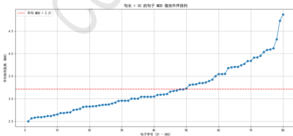
Figure 3: VTB树库句长= 20 时单个句子MDD 升序排列图
