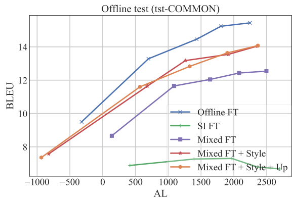
(b) BLEU
