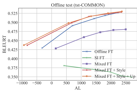
(a) BLEURT
