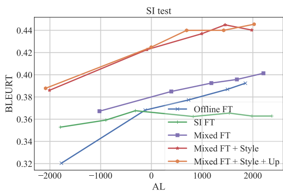
(a) BLEURT
