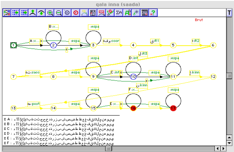
Figure1 : l'automate « qala inna »
