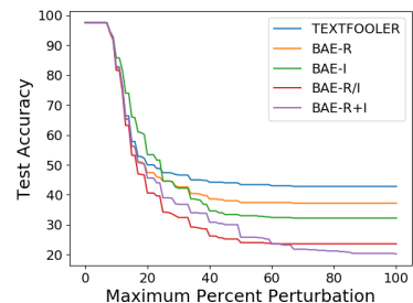
(b) BERT
