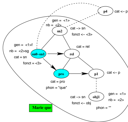
Figure 4: Vue partielle de la description syntaxique D_1 résultant d'une opération de neutralisation élémentaire sur D_0
