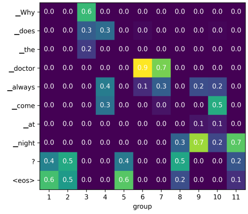
(d) Latent Selecting
