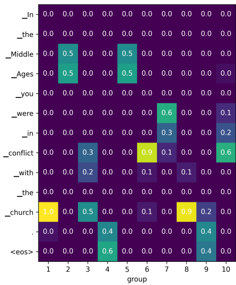
(d) Latent Selecting
