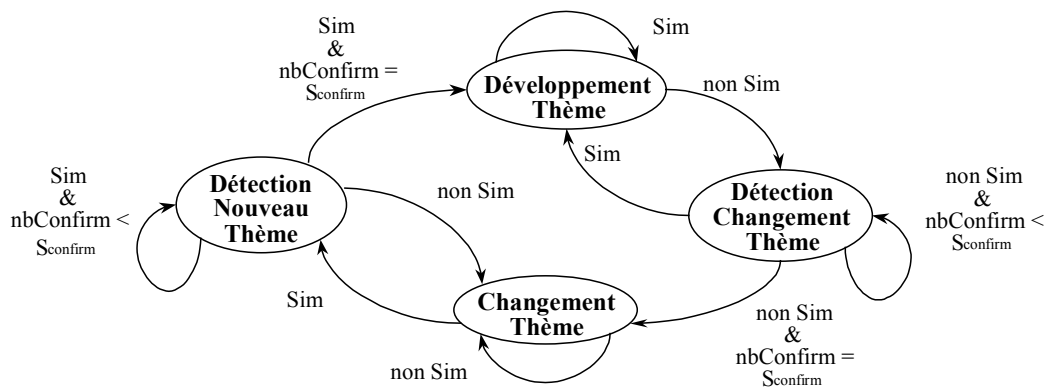
Figure 2 : L'automate de détection des changements de thème
