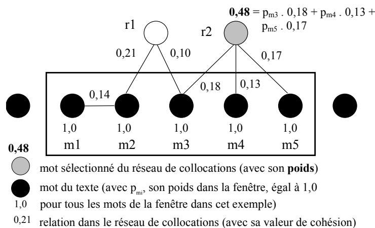
Figure 1 : Sélection et pondération des mots du réseau de collocations
