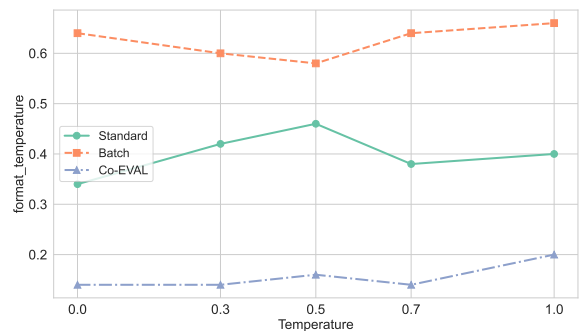
(d) Format
